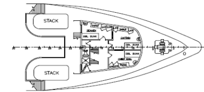
FOCS'L DECK
